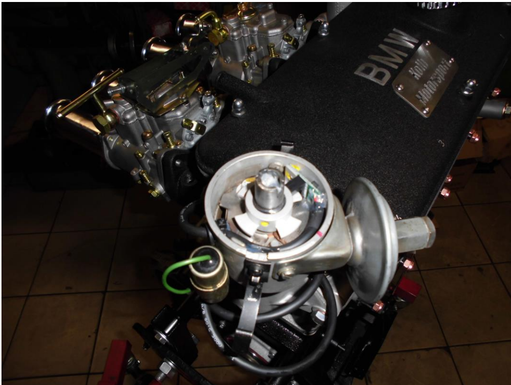
BMW 1800 TISA Kennfeldzündung im Original-Verteiler
